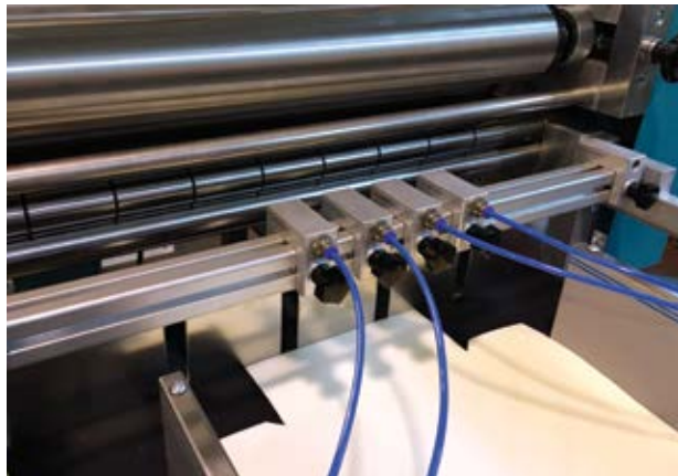
HF Mettifogli per carta anche sagomata e per cartone
